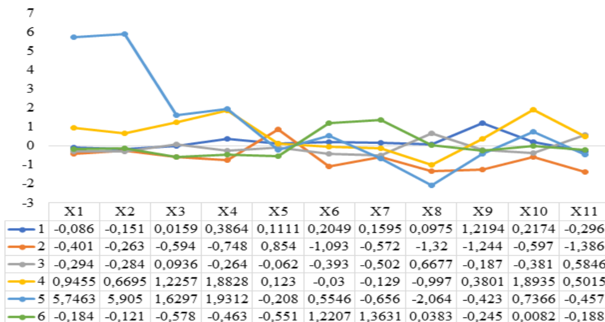
Рисунок 5 – Графическое изображение средних значений для использования метода К-средних 5
